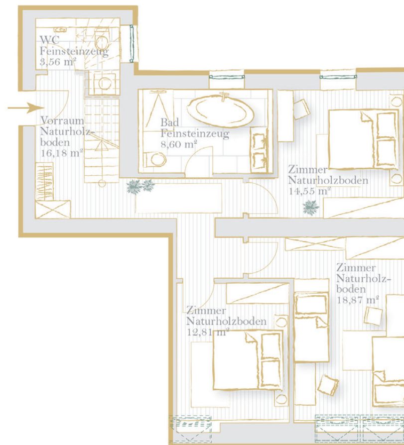
ETAGE IV
